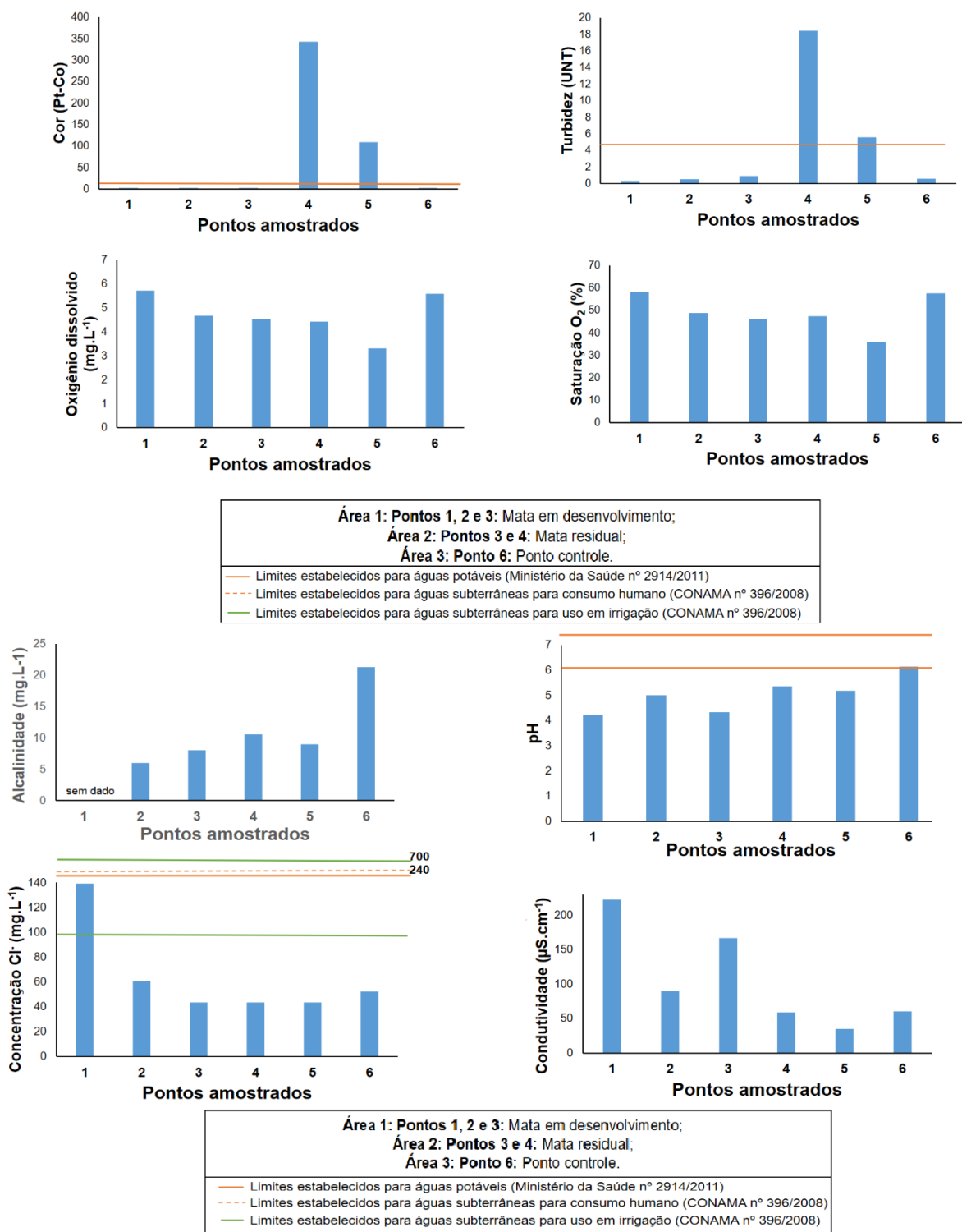
Figura 5 - Resultados da alcalinidade, pH, cloretos e condutividade da água subterrânea de 3 áreas da Ilha dos Marinheiros (Rio Grande/RS)
